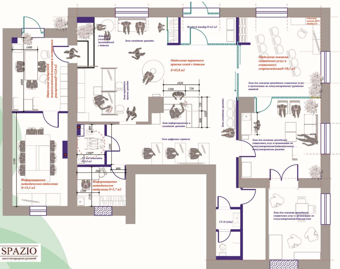
План помещений М 1:50
